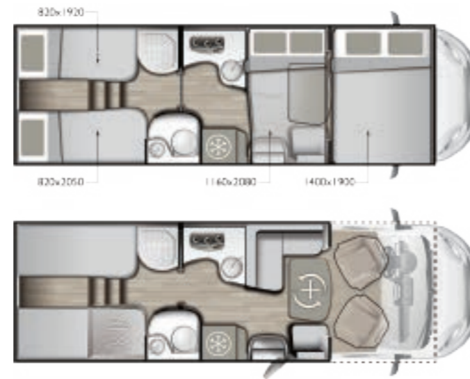
KEA M76 // 7,32 MT
