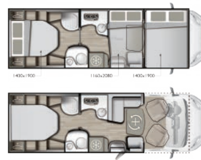
KEA M79 // 7,38 MT
